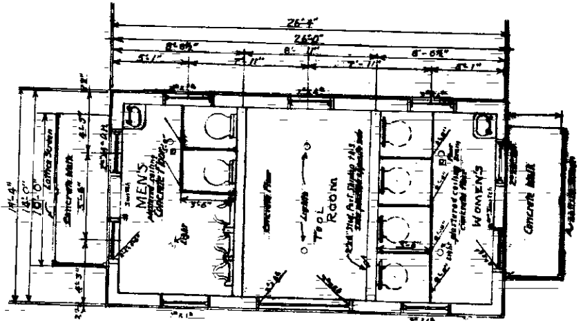
PLAN Scale 1/4\"/>
