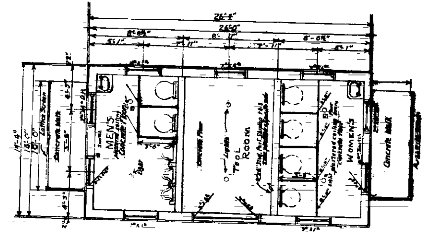
PLAN Scale 1/4\"/>
